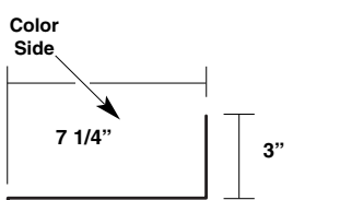
Rake Tie-In Flashing Item #: 38432
